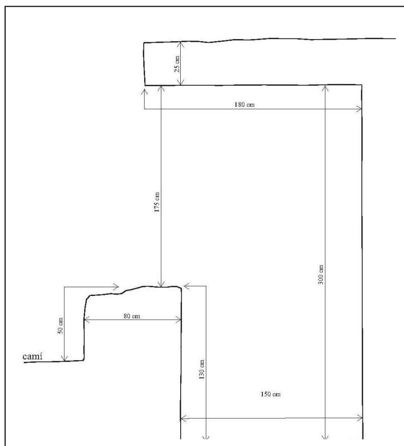
Planta i secció extretes de PÉREZ SUÑÉ, J.M., RAMS FOLCH, P., Neteja i documentació de les fonts, pous i mines a l'entorn del Perelló , Servei d'Arqueologia, 2015. Informe inèdit.
