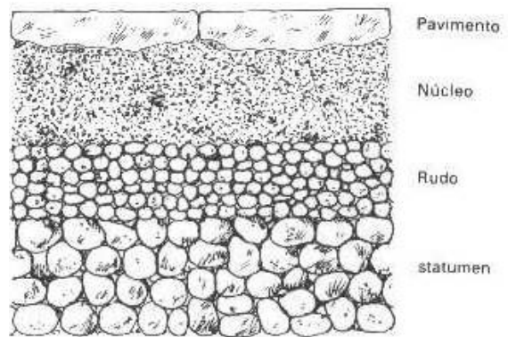
Imatge 4. Estratigrafia d'una via romana. Font: Pàgina web IES Alicante.
