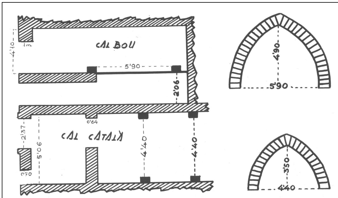
Planta i alçat de BOYER GIL, A., PALLARÈS LLEÓ, A., Història d'El Perelló , volum I, Barcelona 1978, 182.
